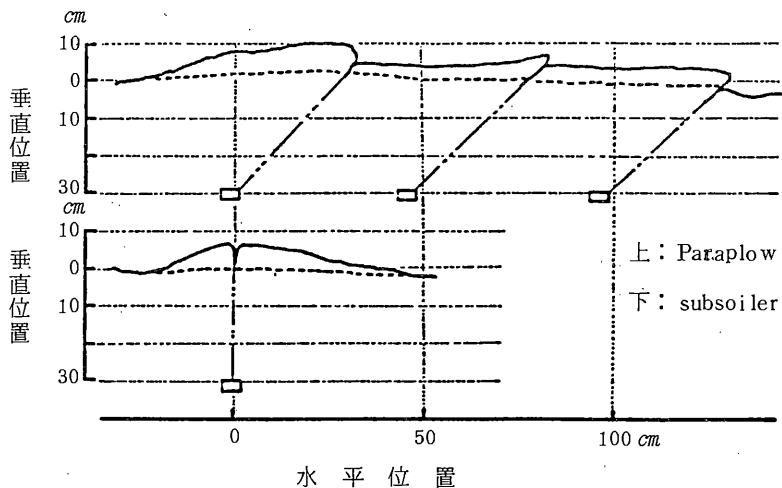
図2. Paraplowとsubsoiler施工後の草地のプロフィール
