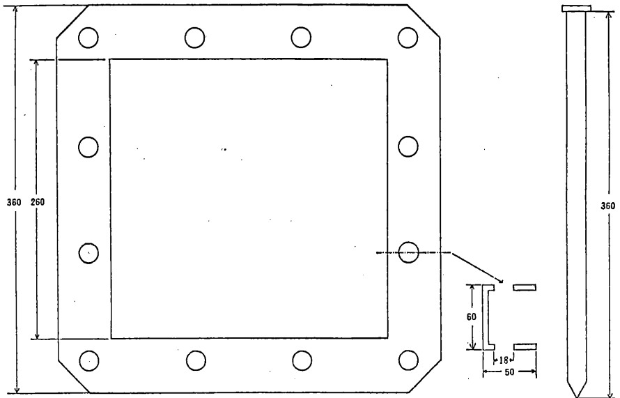
図 2. cubic sampler (単位mm)
