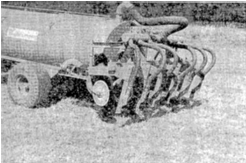
図2. 作土処理スラリインジェクタ — インジェクタの部分为国産化、施工深20cm、巾45cm —
