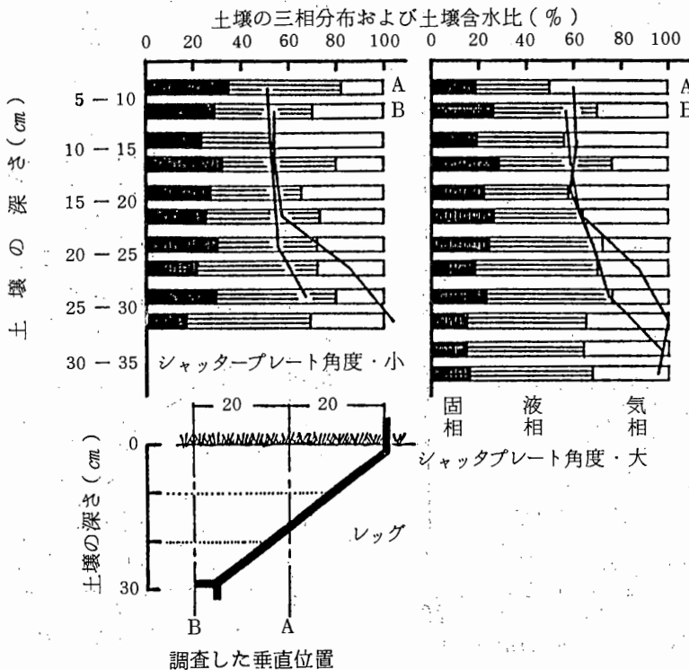
図4. Paraplowの作用部と土壌の三相分布および土壌含水比
