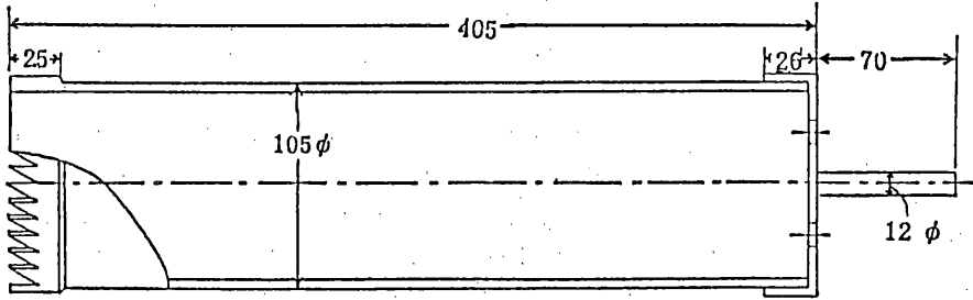
図1. core sampler (単位mm)
