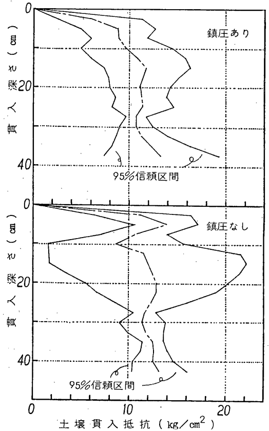
図6. サブソイラ土壌硬度の変化と鎮圧ローラの影響（対照機）
