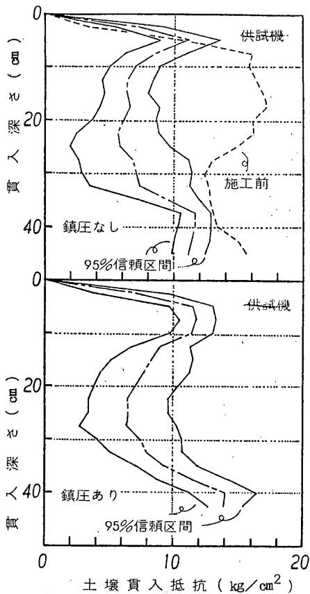
図5. パラプラウ土壌硬度の変化と鎮圧ローラの影響
