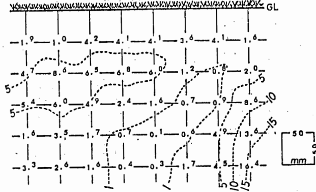
図3. 施工後の土壌硬度の分布(山中式硬度計の指標硬度: mmからSR-2型-小コーン-の貫入抵抗: Kg/cm 2 に換算)
