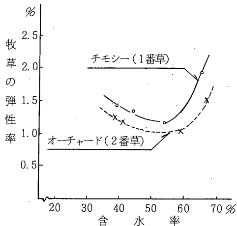
図2. 牧草の含水率と弾性率の関係
