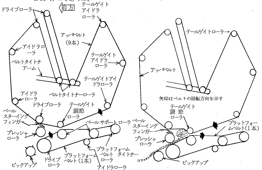
図3. ベルトローラ概略図
