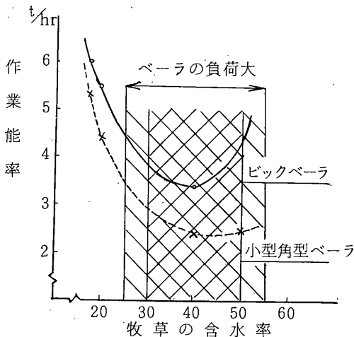
図1. ビッグベールと小型角型ベールの能率と牧草の含水率の関係
