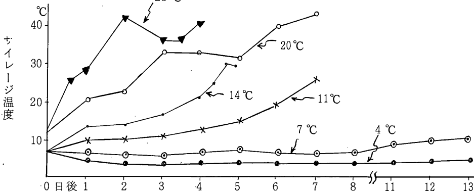
図2. 外気温と変敗の速さ (対照サイレージを供試)
